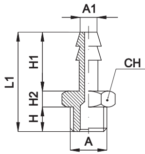
BSP адаптер для трубки
