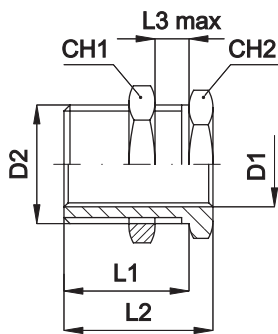
Муфта с внутренней резьбой
