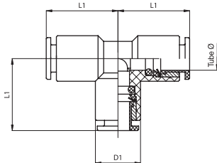
Равноценный тройник
