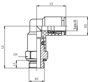
BSP удлиненный поворотный угловой Корпус из полиформальдегида Болт из никелированной латуни с уплотнением OR
