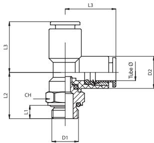
BSP поворотный боковой тройник Корпус из полиформальдегида Болт из никелированной латуни с уплотнениями OR
