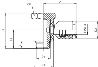
Болт с серьгой угловой Корпус серьги из полиформальдегида Болт из никелированной латуни
