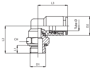
BSP поворотный угловой Корпус из полиформальдегида Болт из никелированной латуни с уплотнением OR
