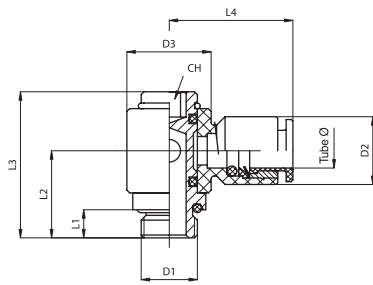
BSP угловой с гайкой Корпус из полиформальдегида Болт из никелированной латуни с уплотнением OR
